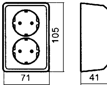
Målskisse
